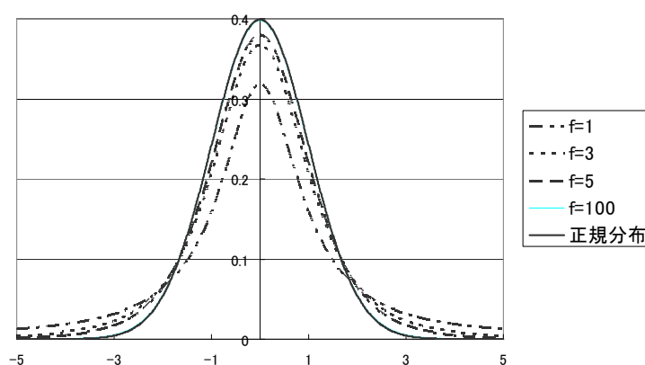
図 t 分布と正規分布（ n=\infty のとき t 分布は正規分布と一致する）
