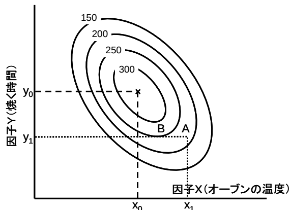
図 2 2 因子応答曲面の等高線図
