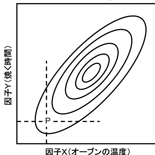
図3 最適な水準に到達しない実験例
